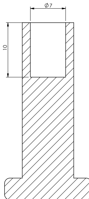
SECTION A-A SCALE 3 : 1
